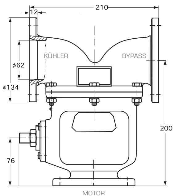
Typ X3.250.*)1.000, Seitenansicht
