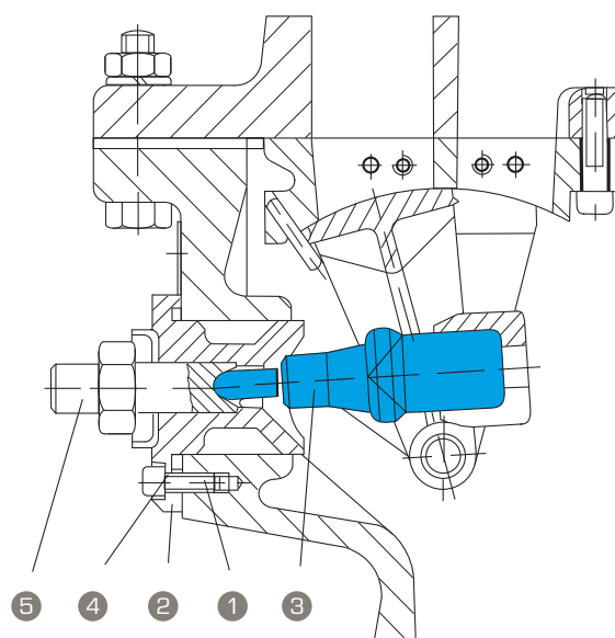
Typ X3.250.*)1.000, mit Dehnstoffarbeitselementen-Schwinge
